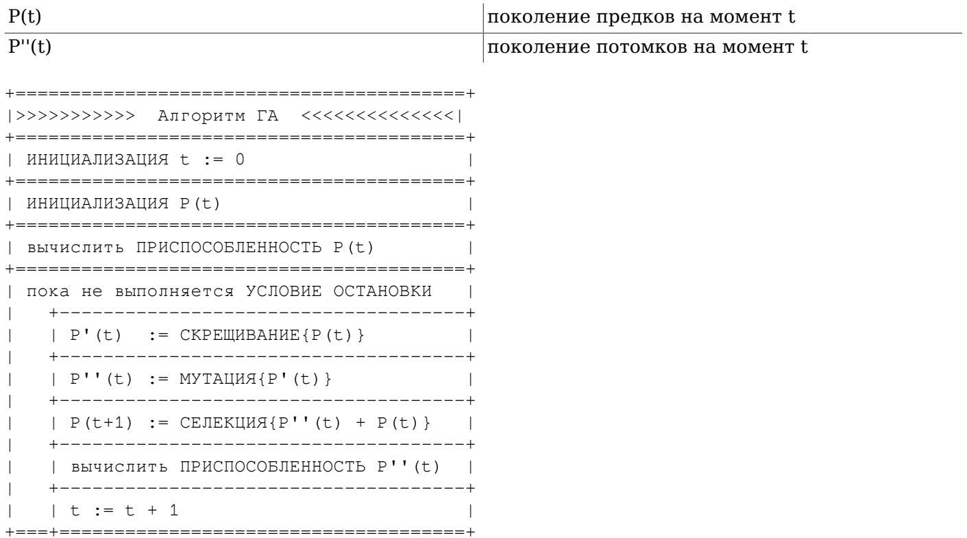
Рисунок 58.1. Диаграмма структуры генетического алгоритма
