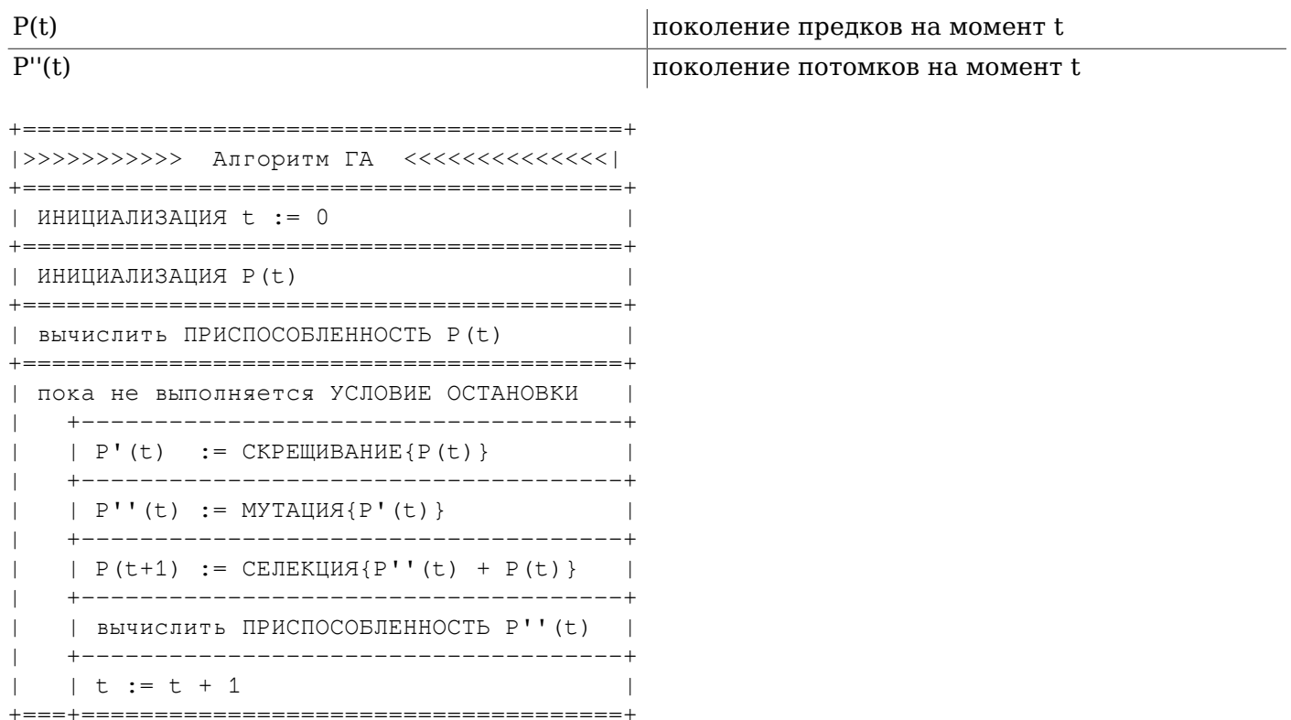
Рисунок 55.1. Диаграмма структуры генетического алгоритма
