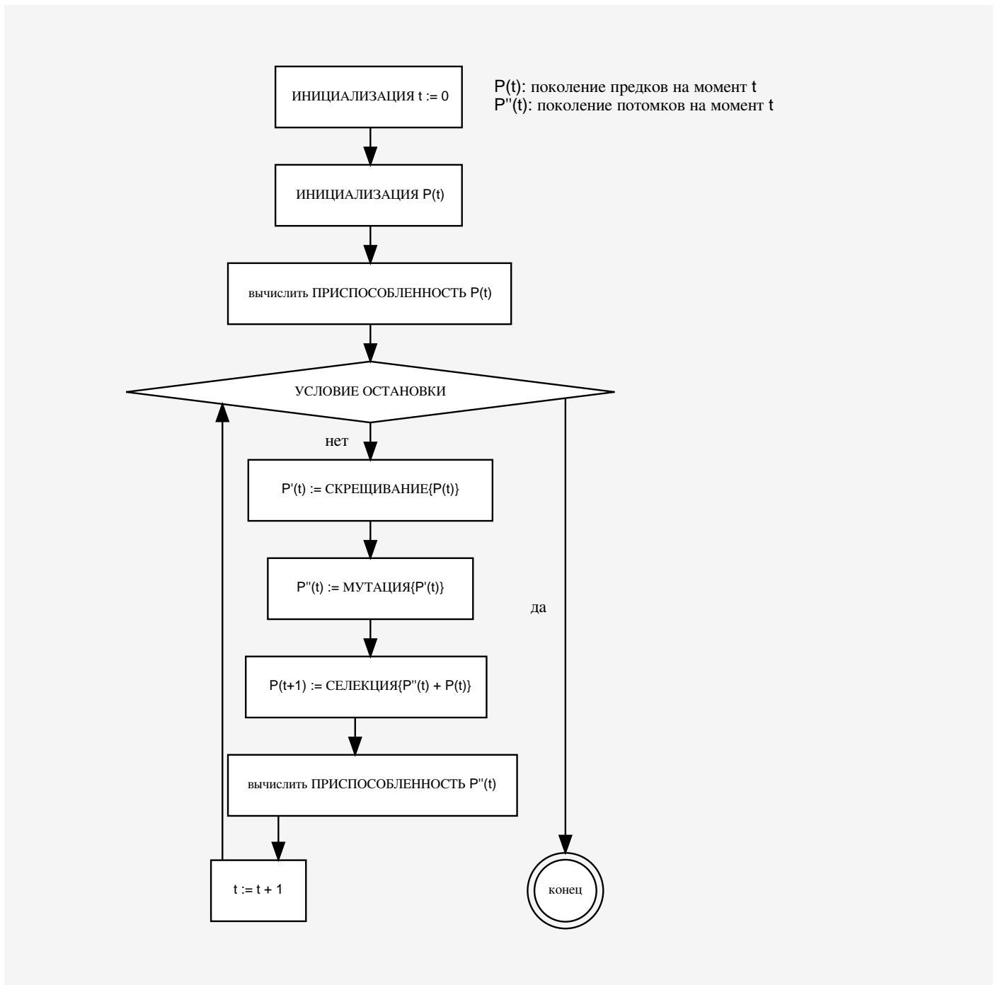
Рисунок 56.1. Структура генетического алгоритма
