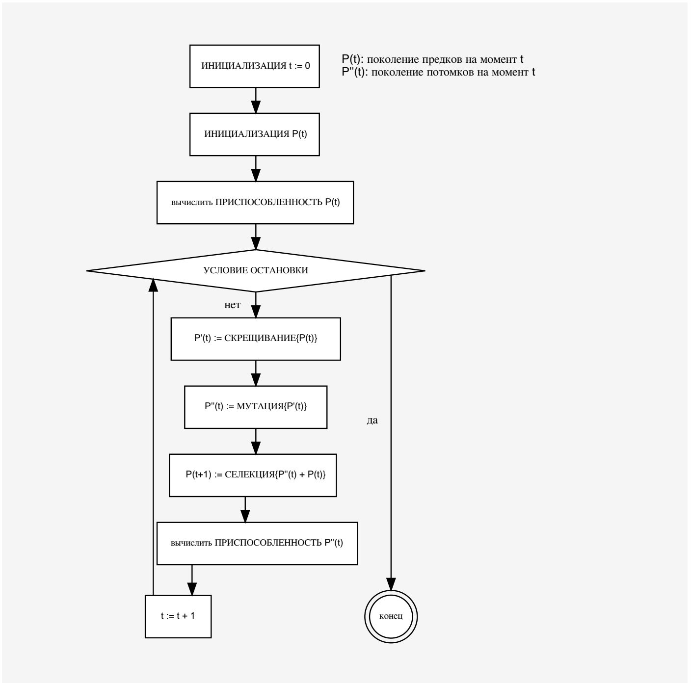
Рисунок 61.1. Структура генетического алгоритма
